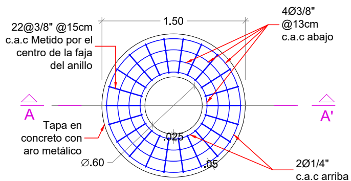
PLANTA DISTRIBUCIÓN DEL REFUERZO
