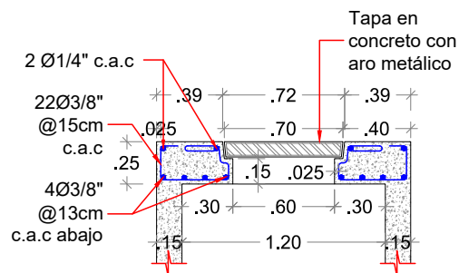
CORTE DE LOSA
